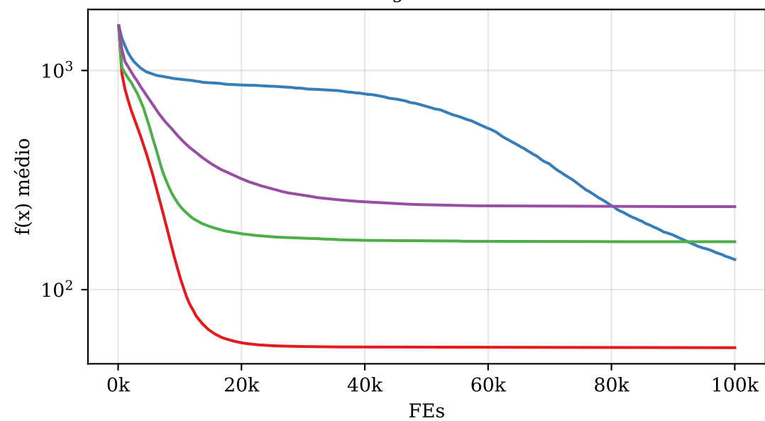
Schwefel 2.26 — D=100
