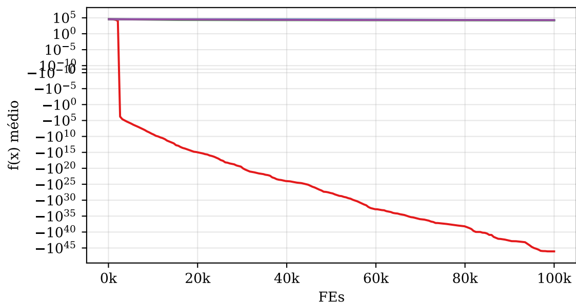
Schwefel 2.26 — D=100
