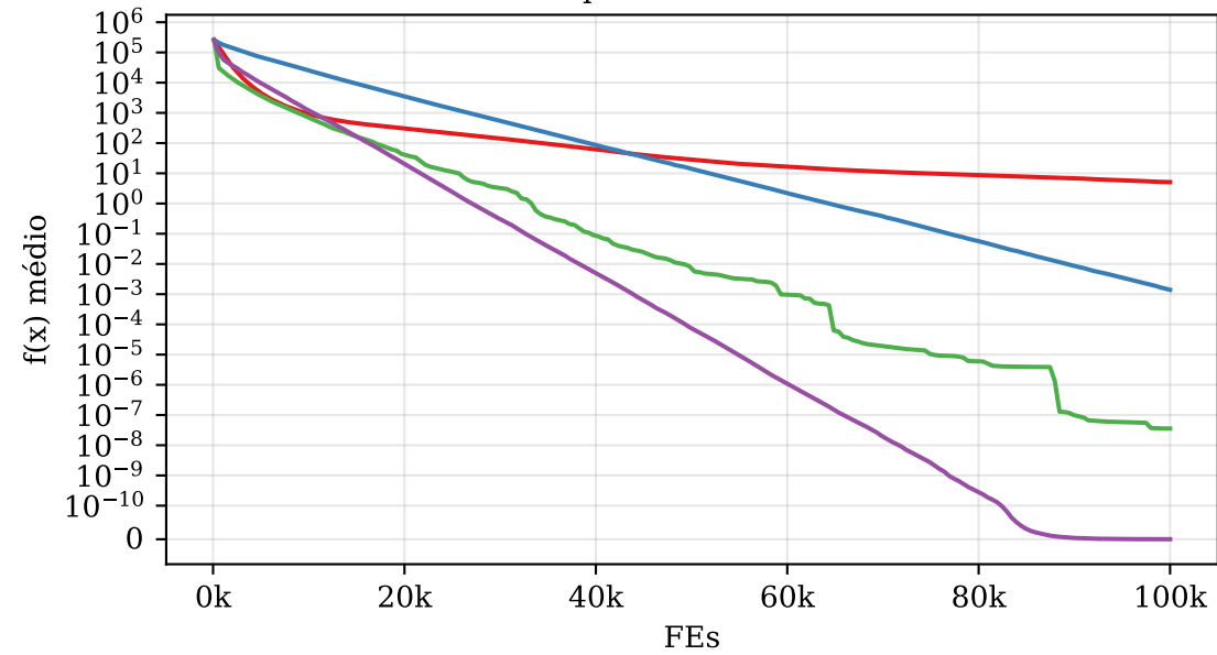
Rosenbrock — D=100
