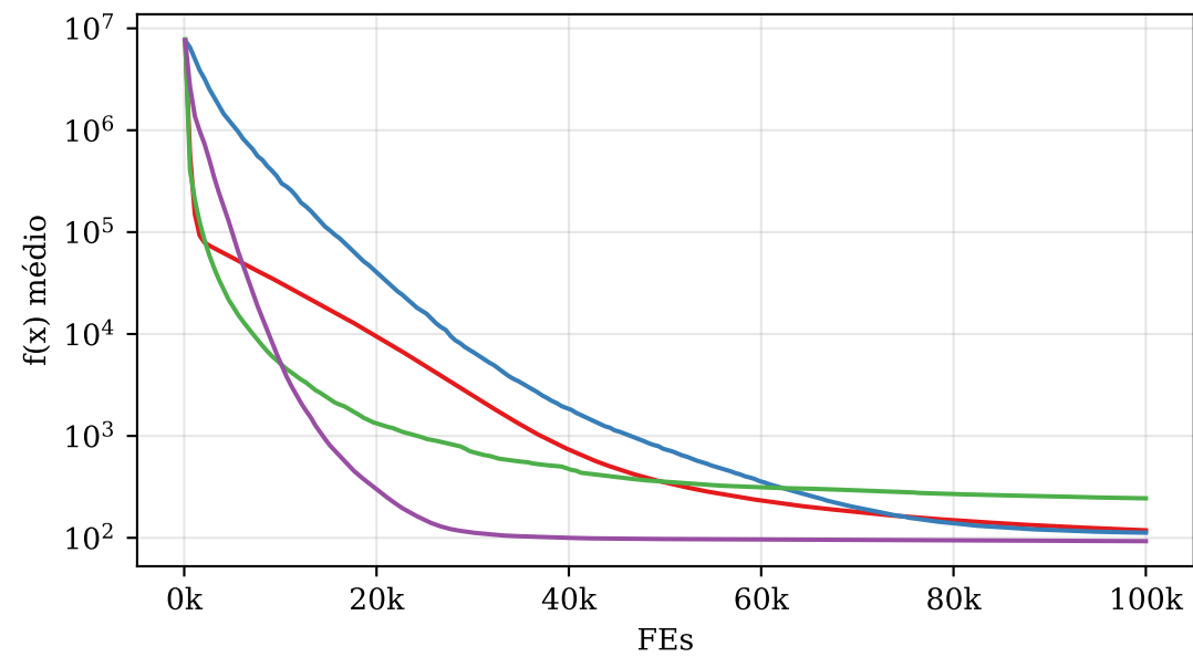
Rastrigin — D=100
